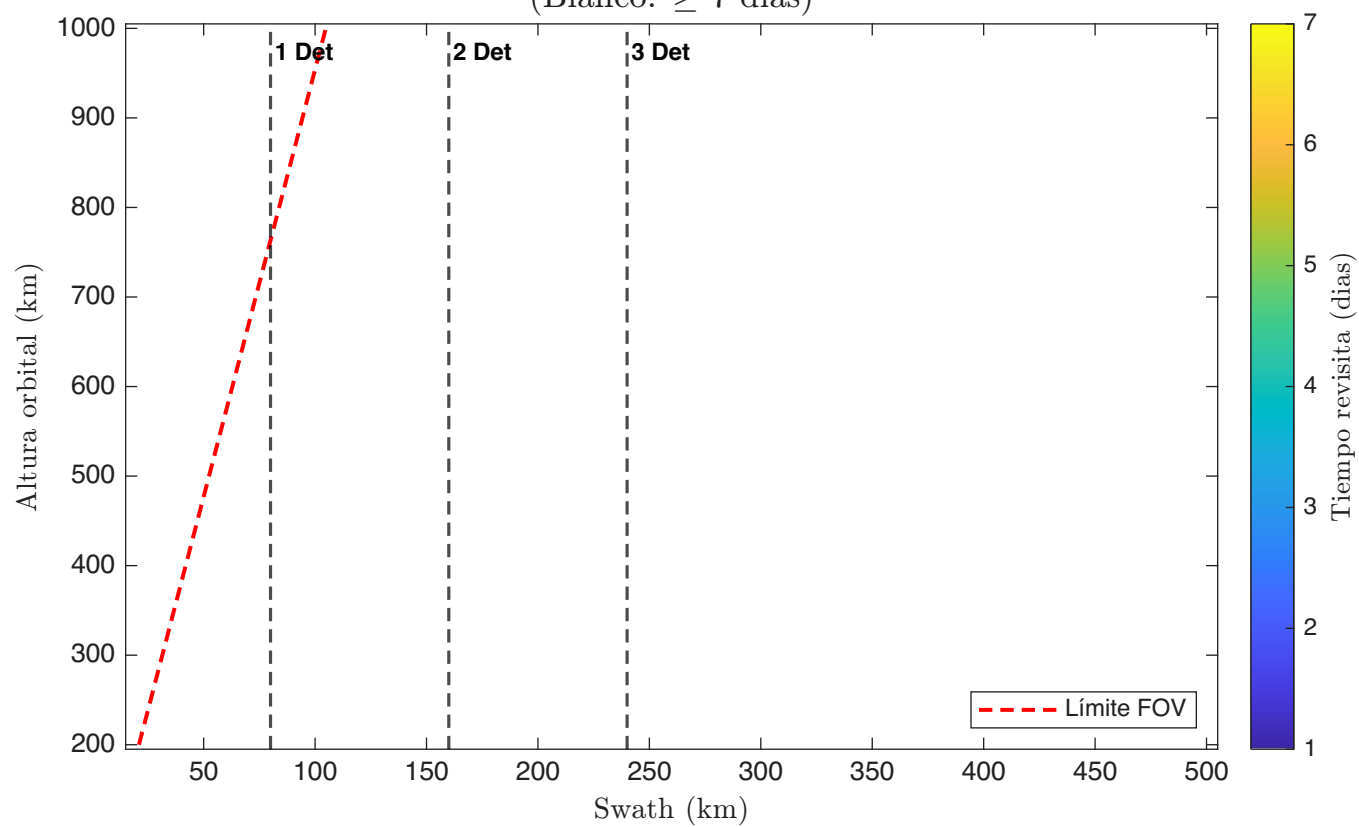
Tiempo Revisita - 1 Satellite(s); 2 Telescopio(s): Korsch; Detector 3 (Blanco: \geq 7 dias)
